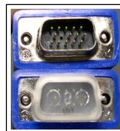
VGA ケーブルのピン形状 （下はカバー付きの状態）
